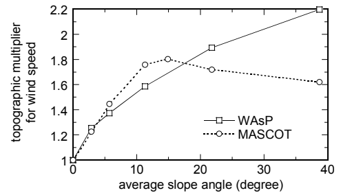
図3 山頂での風速比の傾斜角度による変化
