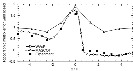
図2 風速比の流れ方向の変化
