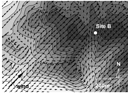
図5 B地点SW風向における地上10mでの風速ベクトル
