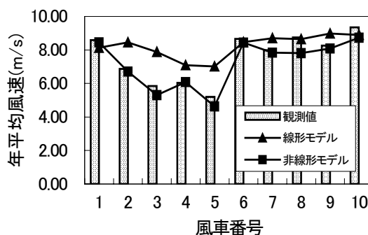
図11 年平均風速の予測結果と観測値との比較
