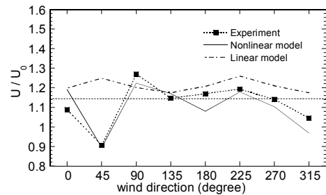
図8 F地点での地上40mにおける風向別風速比
