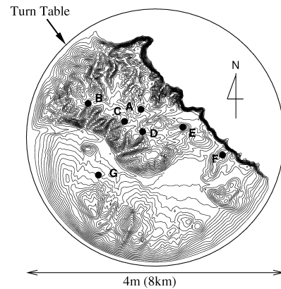
図4 地形の等高線と測定点の配置
