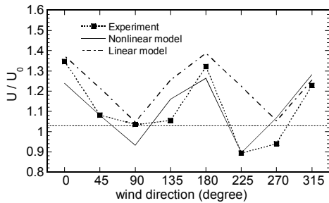
図6 B地点での地上40mにおける風向別風速比
