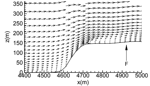
図7 F地点NE風向における垂直断面内の風速ベクトル
