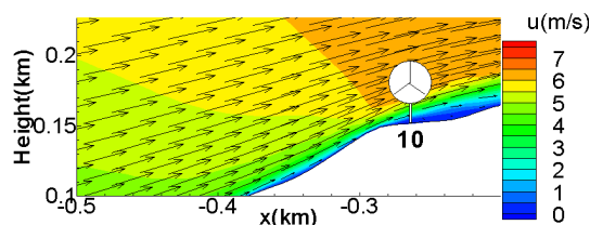
図10 E-W断面内の平均風速ベクトル(上:5号機下:10号機)
