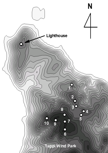
図9 竜飛ウインドパーク内の風車の配置図
