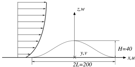
図1 2次元尾根の形状 (平均傾斜角 21.8度)
